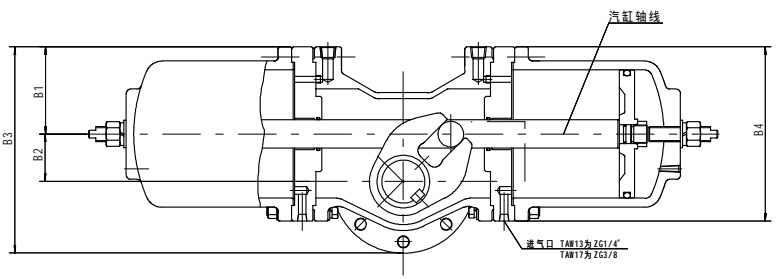
TAG, TAW 连接型式尺寸
